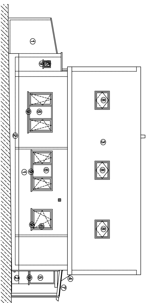
linker zijgevel
